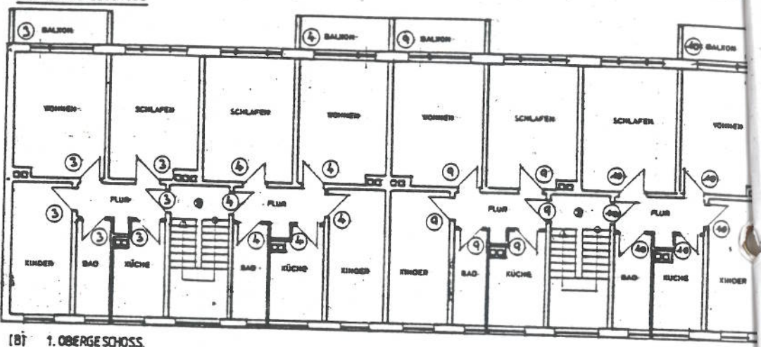
[B] 1. OBERGESCHOSS
